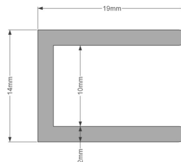
Muurprofiel/profilé mural
