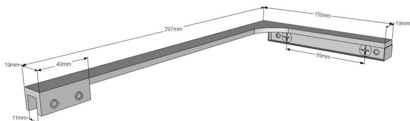
Stabilisatie/stabilisation (lengte/longueur 297/447mm)
