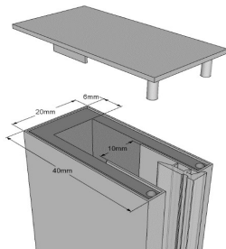
Muurprofiel draaideur / profilé mural porte
