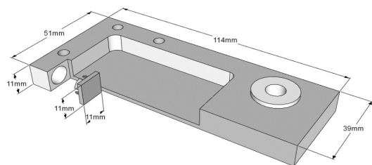
Pivot stuk op grond / Pièce de pivot au sol
