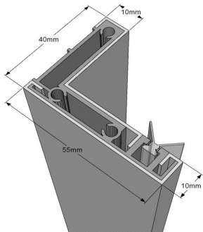
Waterkeringsprofiel / Profilé d'échanchéité
