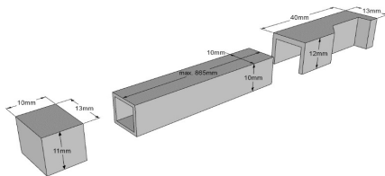
Waterkeringsprofiel / Profilé d'échanchéité
