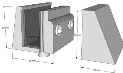
Pivot stuk op glas / Pièce pivot sur le verre
